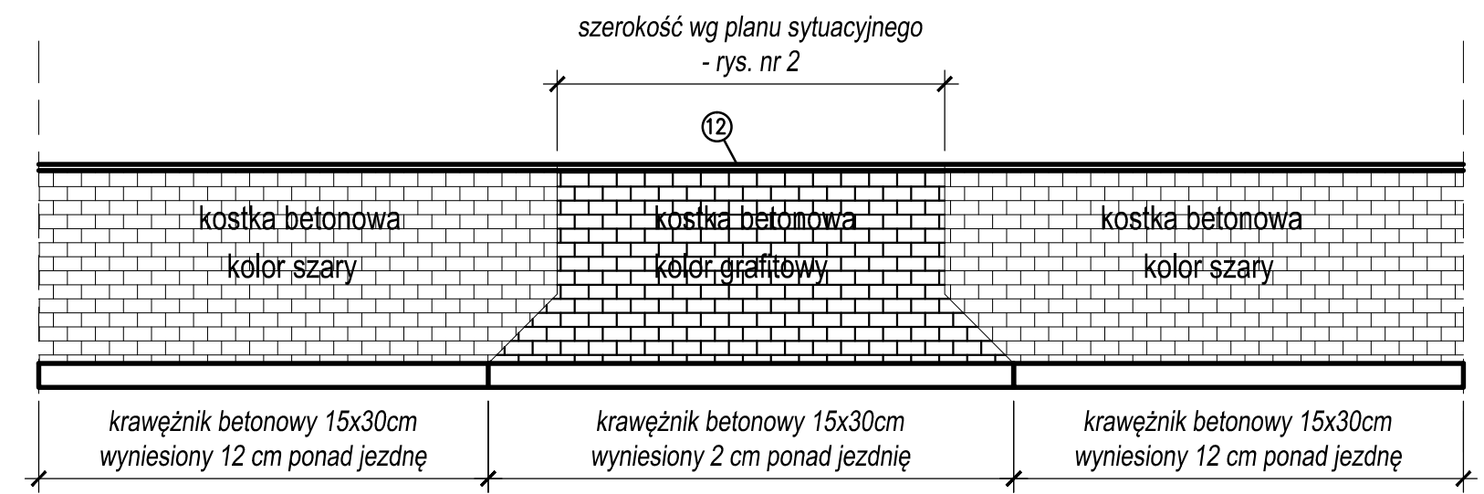
Schemat zjazdu przez ścieżkę pieszo – rowerową
