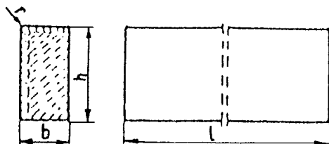
Rys. 1. Wymiarowanie krawężnika betonowego rodzaju b.
